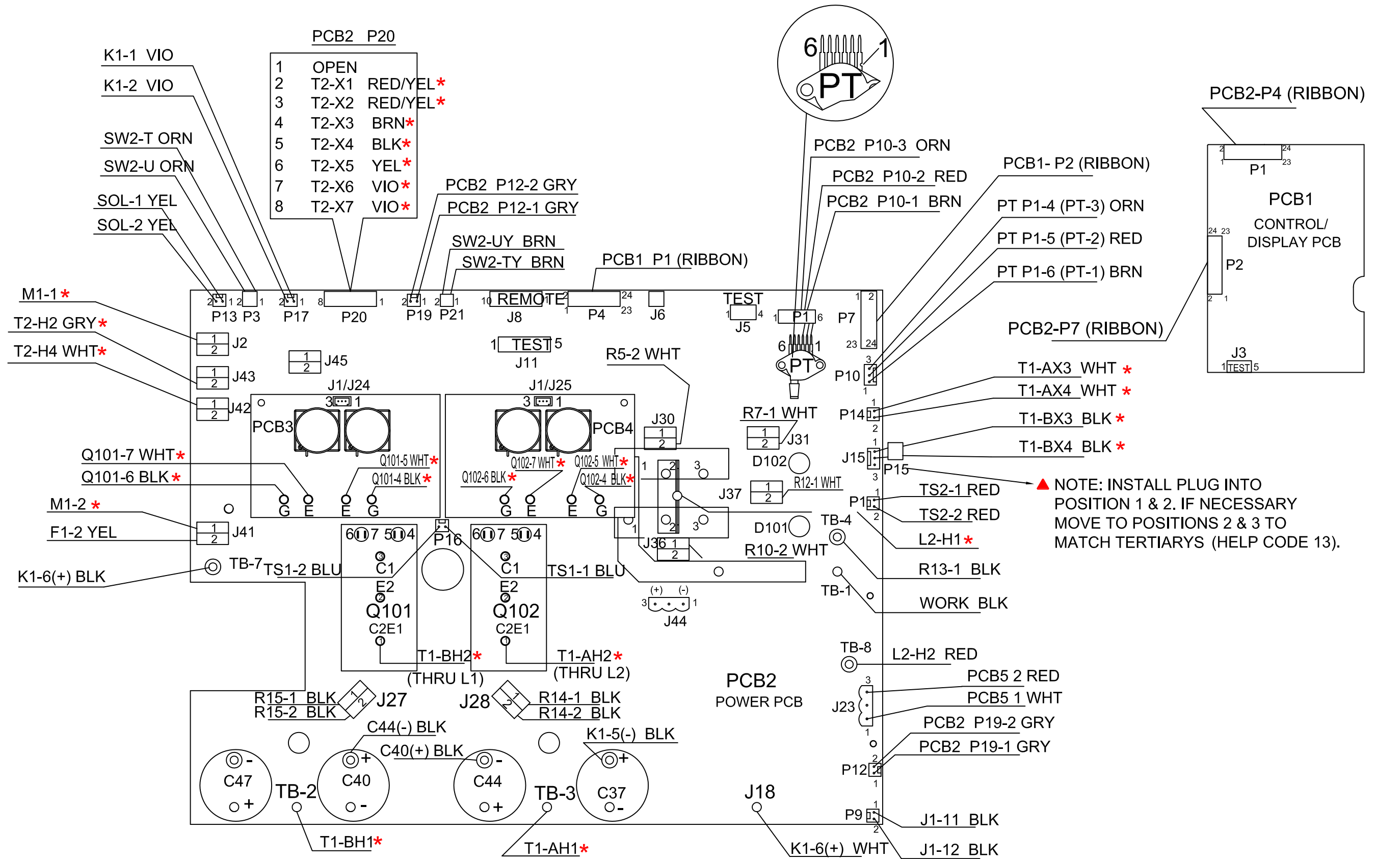
5.3 Wiring Diagram 575V (0558007545)
