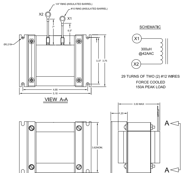
Input Inductor 0558007151
