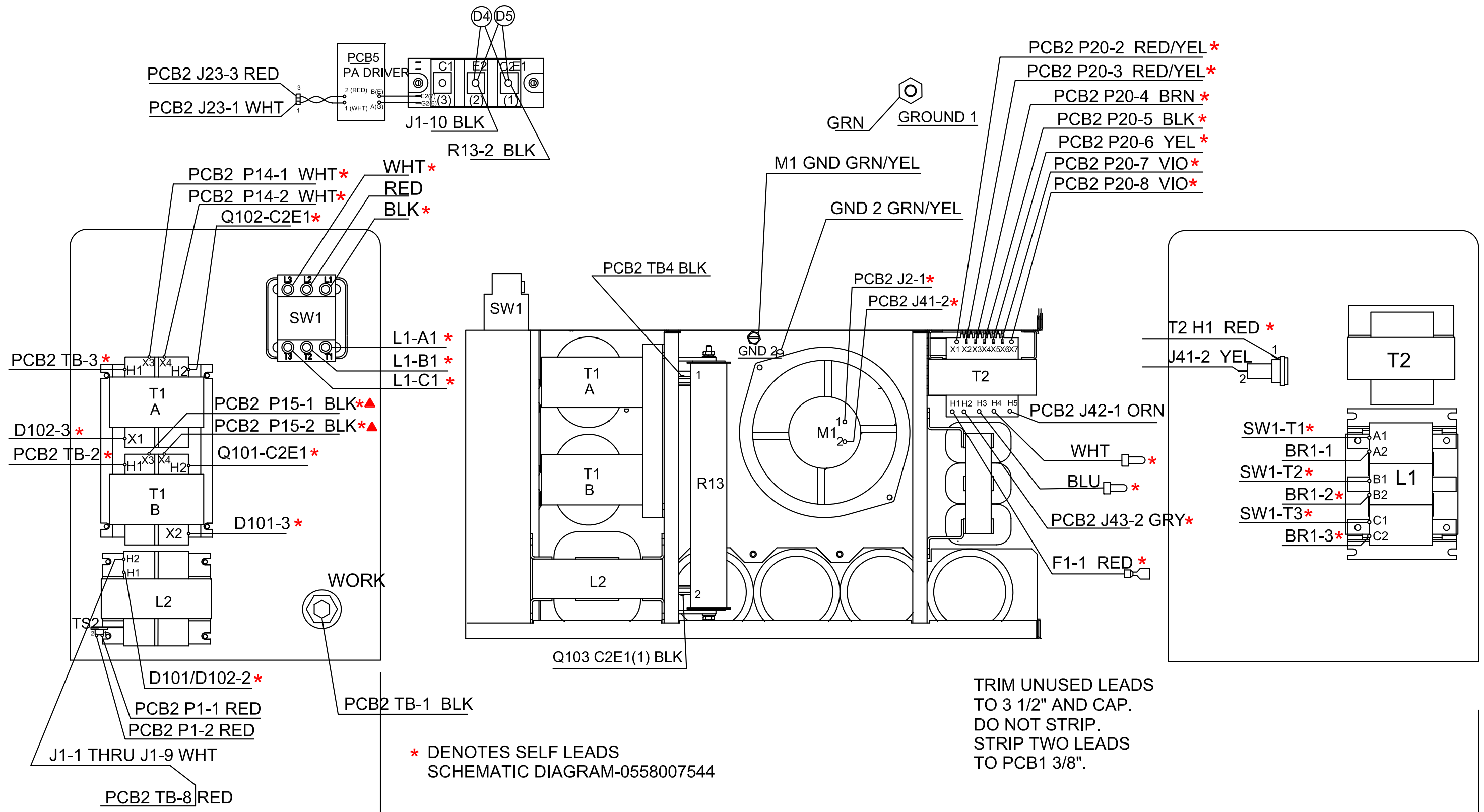
5.3 Wiring Diagram 575V (0558007545)
