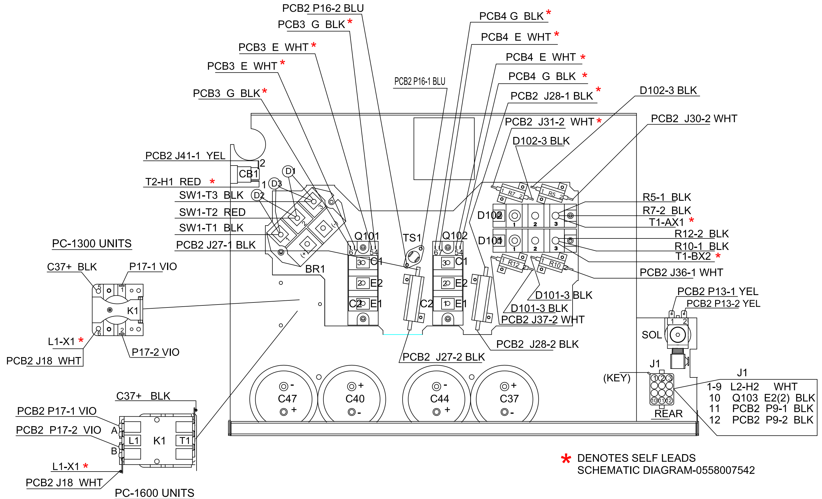
5.1 Wiring Diagram 230/460 Volt (0558007543)
