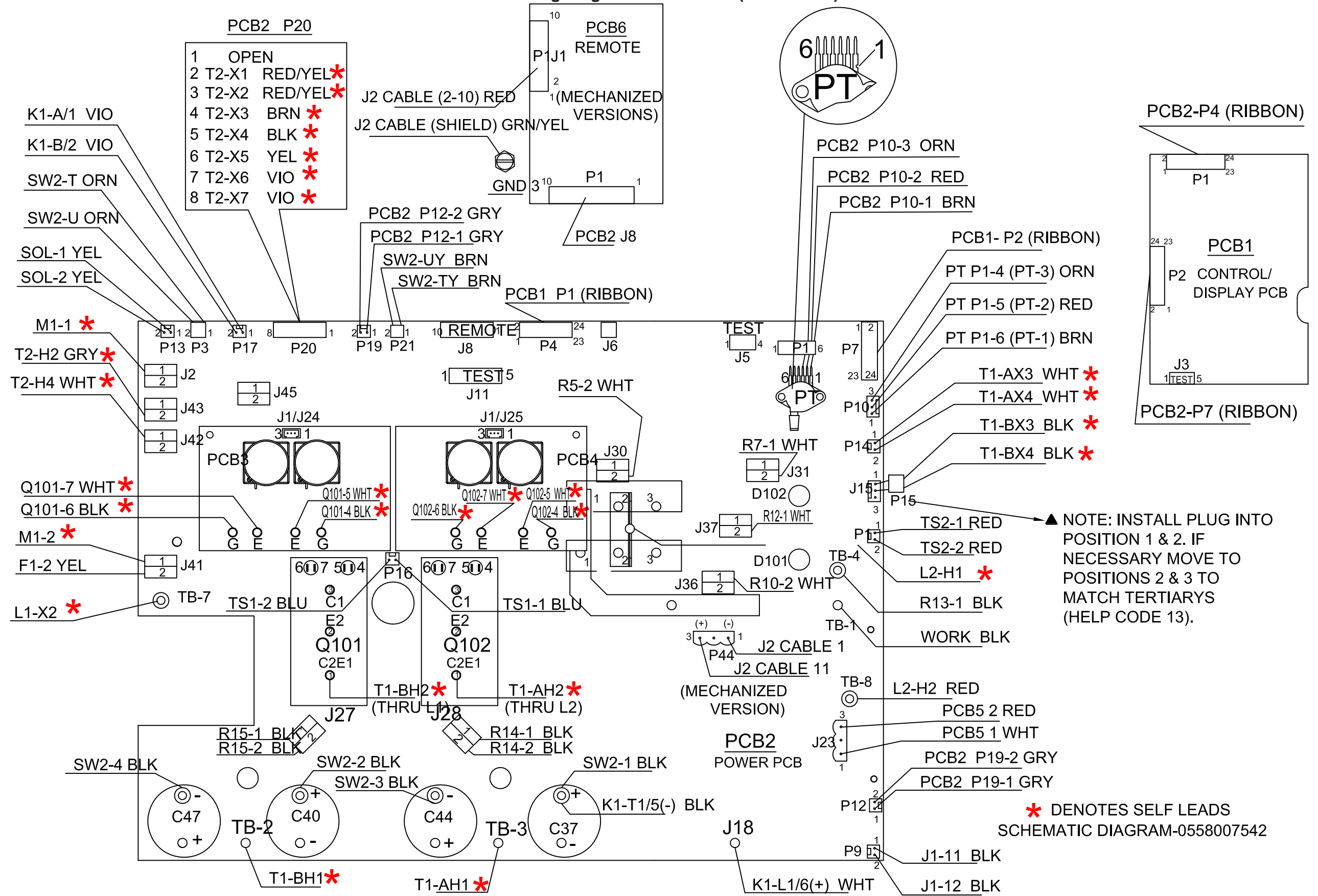
5.1 Wiring Diagram 230/460 Volt (0558007543)
