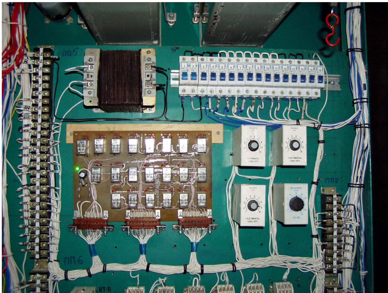
Рис.2 Внешний вид автоматики безопасности и розжига парового котла
