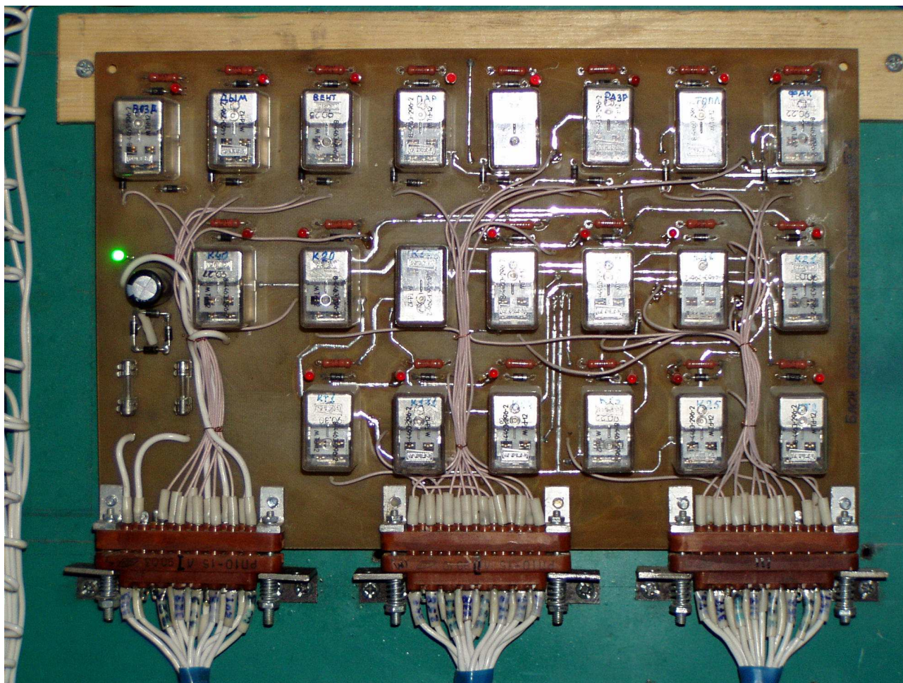
Рис.2 Внешний вид релейного блока автоматики безопасности и розжига парового котла
