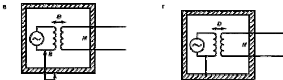
Защита между первичными опасными для жизни цепями и доступными клеммами вторичных цепей, в которых не превышены значения 6.3.1 в нормальных условиях Рисунок D.2, лист 2
