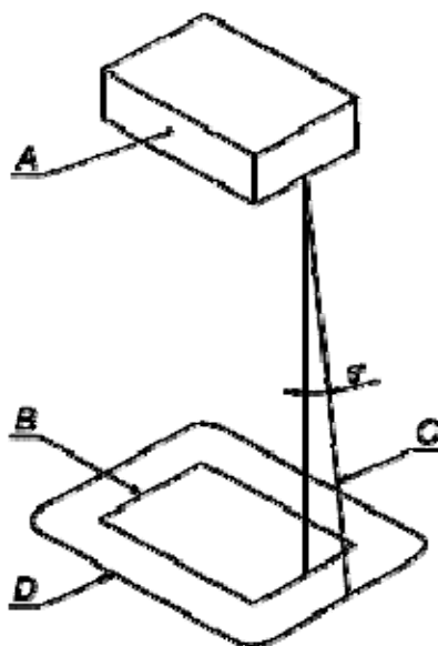
A - часть или компонент оборудования, который рассматривают как источник опасности от огня. Это компонент в целом или часть оборудования, если она не защищена другим способом, или же незащищенная часть компонента, который частично защищен своим корпусом; B - проекция контуров части A на горизонтальную плоскость; C - наклонная линия, которая очерчивает минимальную зону основания и расположение боковых сторон, которые должны быть выполнены в соответствии с требованиями 9.2.1, перечисления б) 1) и б) 2). Эту линию проводят под углом 5^\circ от вертикали в каждой точке периметра A и ориентируют таким образом, чтобы занять максимальную площадь; D - минимальная зона основания, которая должна соответствовать требованиям 9.2.1, перечисление б) 1) Рисунок 7 - Участок основания кожуха, который сконструирован в соответствии с 9.2.1, перечисление б) 1)
