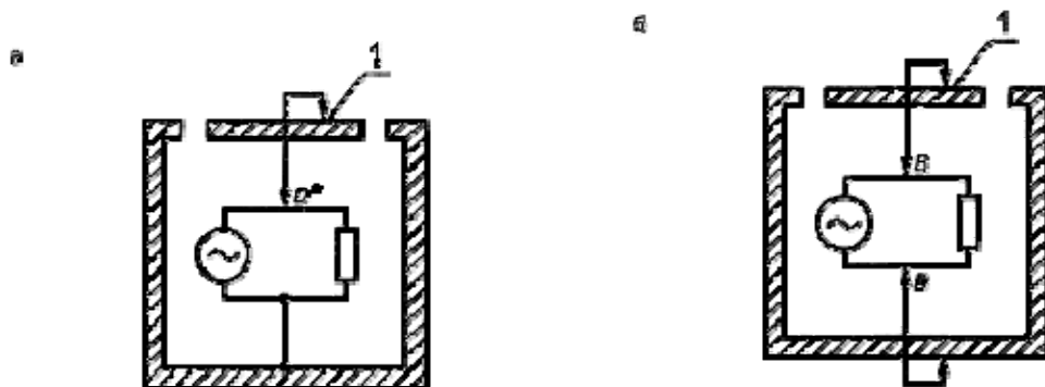
1 - доступная часть, электрически не соединенная с другими доступными частями Защита между внутренними опасными для жизни цепями и доступными частями, которые электрически не соединены с другими доступными частями Рисунок D.2, лист 1
