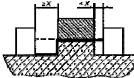
Рисунок С.1, лист 2
