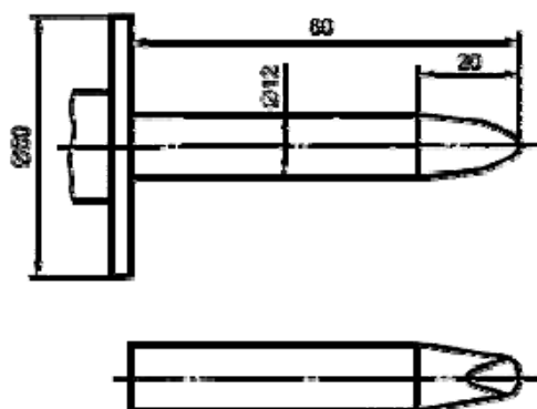
Рисунок В.1 - Жесткий испытательный палец (испытательный шуп 11 по ГОСТ Р МЭК 61032)
