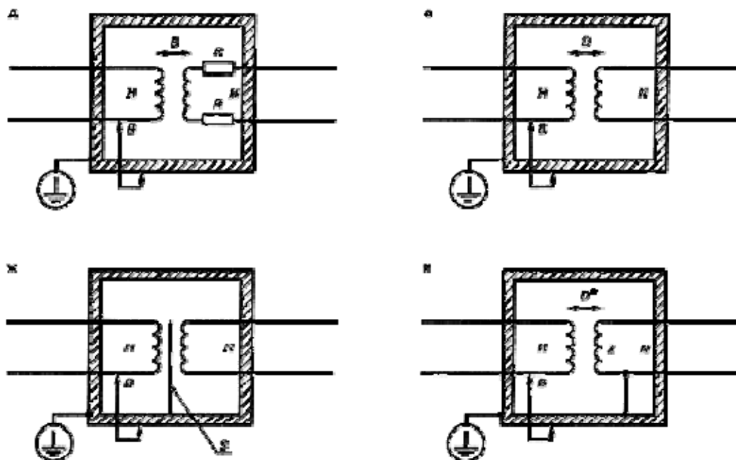
Рисунок D.1 - Защита между опасными для жизни цепями и цепями, в которых не превышены значения 6.3.1 в нормальных условиях и которые имеют внешние клеммы на доступных частях, лист 1
