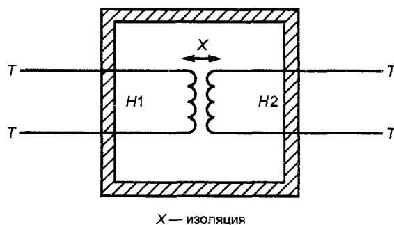
Рисунок D.3 - Защита внешних доступных клемм от двух опасных для жизни цепей
