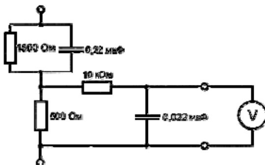
Рисунок А.1 - Схема измерения переменного тока при частотах до 1 МГц и постоянного тока
