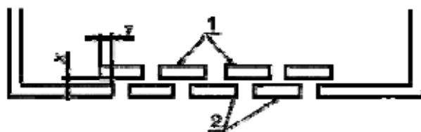
Y - равно удвоенному значению X , но не должно быть менее 25 мм; 1 - полосы перегородки (могут быть ниже основания кожуха); 2 - основание кожуха Рисунок 6 - Перегородки
